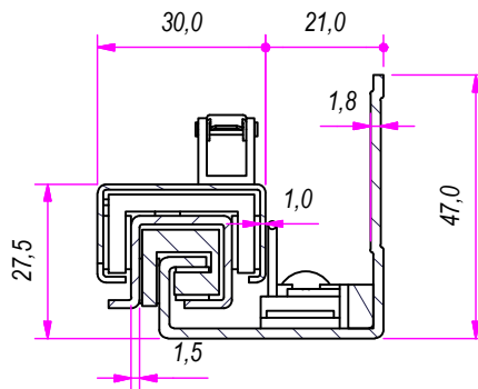
SEZ. A-A
