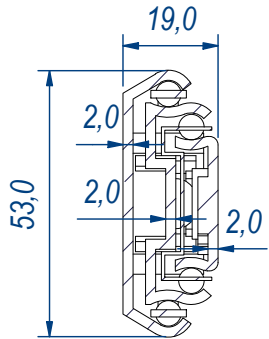
SEZ. A-A
