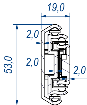
SEZ. A-A
