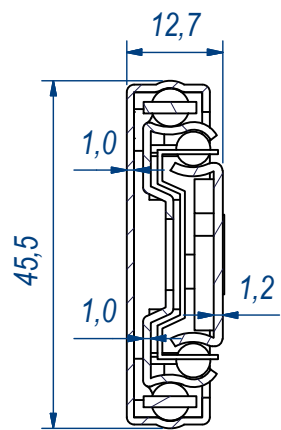
SEZ. A-A
