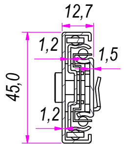
SEZ. A-A
